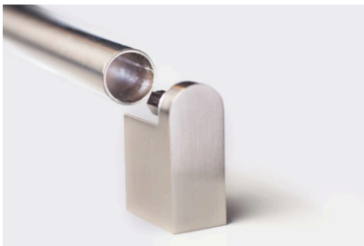
Bildtext: Leichtigkeit und Stabilität müssen einander nicht ausschließen. Das zeigen die neuen Rohrgriffe, die D-Beschlag zunächst für eine Griffserie, die bereits mit massivem Stahl im Programm ist, umgesetzt hat. Foto: D-Beschlag
