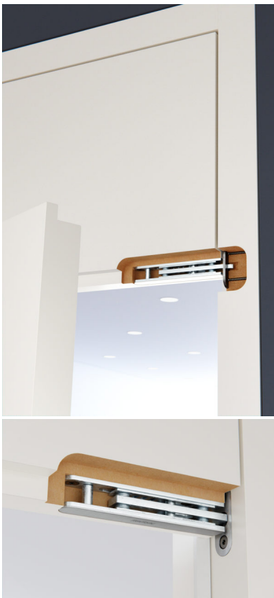
Bildtext: Neben einem herkömmlichen Blendenhalter mit vernickelter Oberfläche und lediglich seitlich verschiebbaren Bauteilen, ergänzt ein dreidimensional justierbarer Blendenhalter aus massivem Stahl das Sortiment von Basys. Foto: Basys
