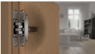
Bildtext: Das „Pivota DX Close“ ist ein verdeckt liegendes Band, das Türen sanft und selbsttätig schließt. Foto: Basys
