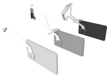
Bildtext 1: Mit der neuen „FREEslim“-Familie gibt Kesseböhmer einen Ausblick auf eine zukünftige Beschlaggeneration im Oberschrankbereich. Dazu gehören „FREEslim fold“ als Klappenfaltbeschlag, „FREEslim slide“ als paralleler Hochschwenk- und „FREEslim swing“ als Hochschwenkbeschlag. Mit nur 8 mm präsentiert sich die Kraftspeichereinheit so flach wie ein „iPad“. Foto: Kesseböhmer
